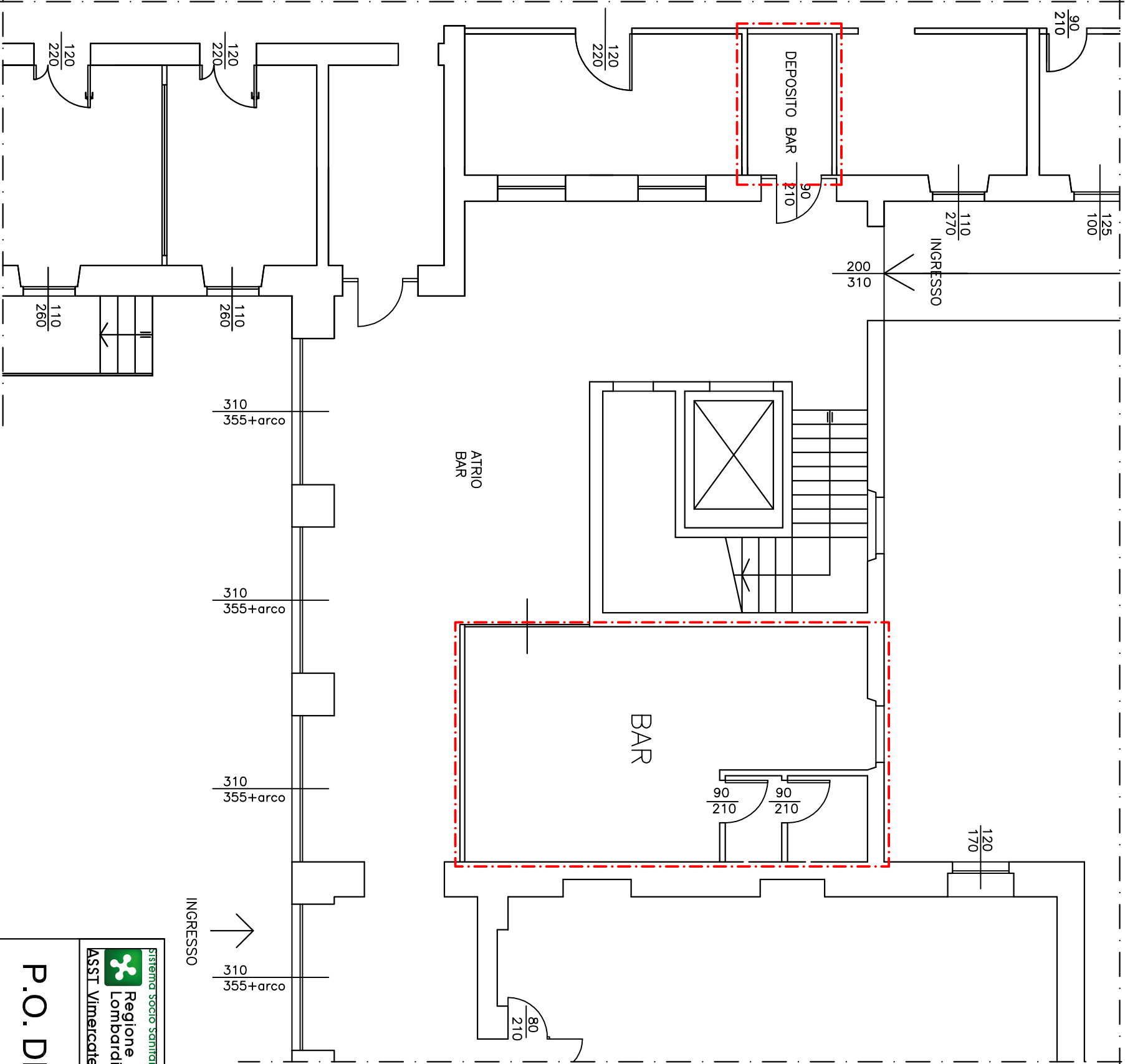
PLANIMETRIA - scala 1:100
